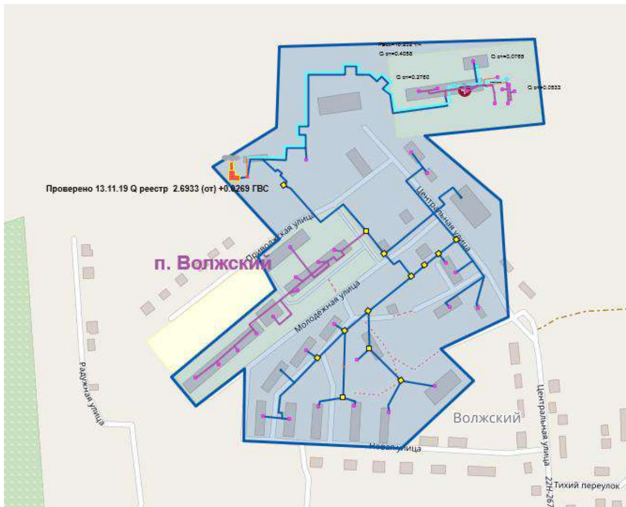
Рис 2.1.1 Зона действия котельной пос. Волжский
