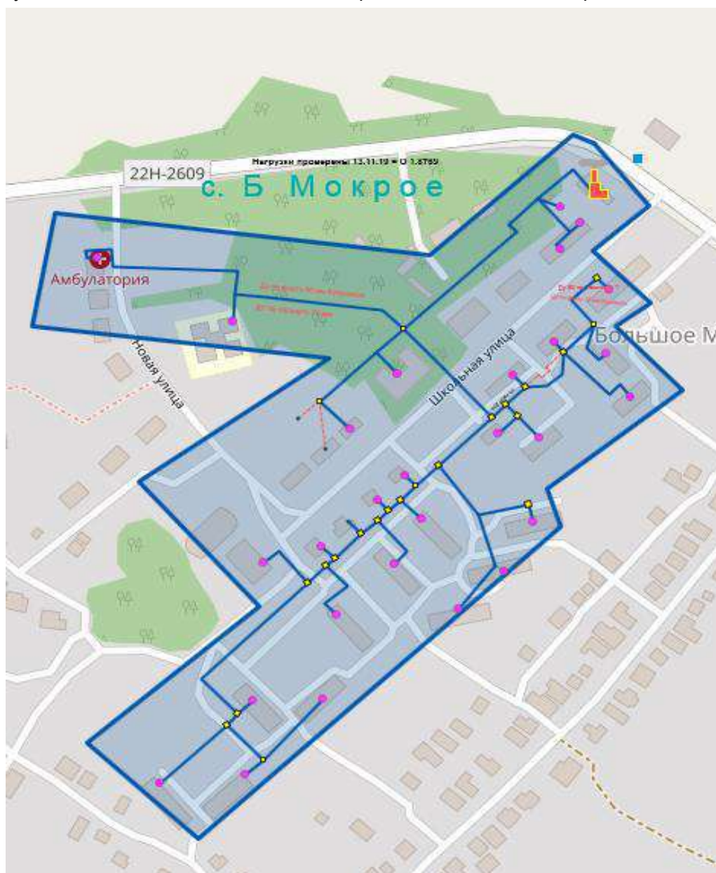
Рис. 2.1.1. Зона действия котельной с. Б. Мокрое
