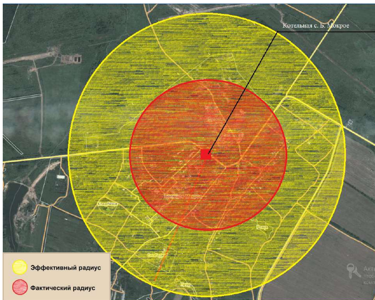
Рис. 2.5.1. Эффективный радиус теплоснабжения котельной с. Б. Мокрое
