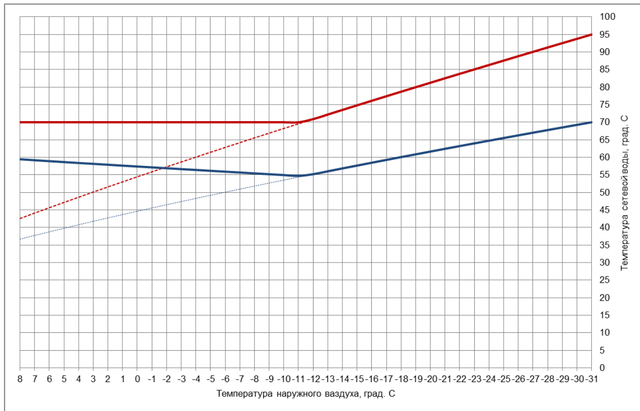
Рис. 5.8.1. Температурный график регулирования для системы теплоснабжения от котельных сельского поселения Большемокринский сельсовет
