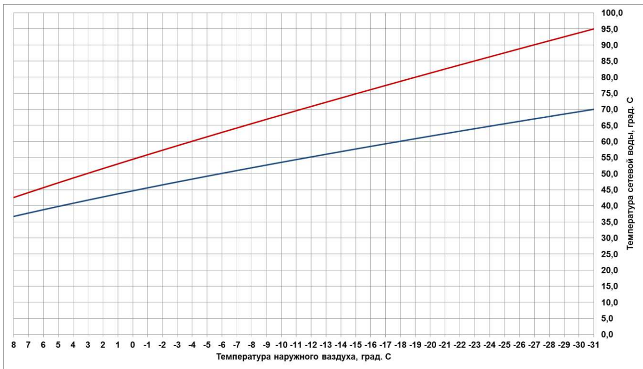
Рис. 4.2.1. Температурный график регулирования для системы теплоснабжения от котельной сельского поселения Безводнинский сельсовет
