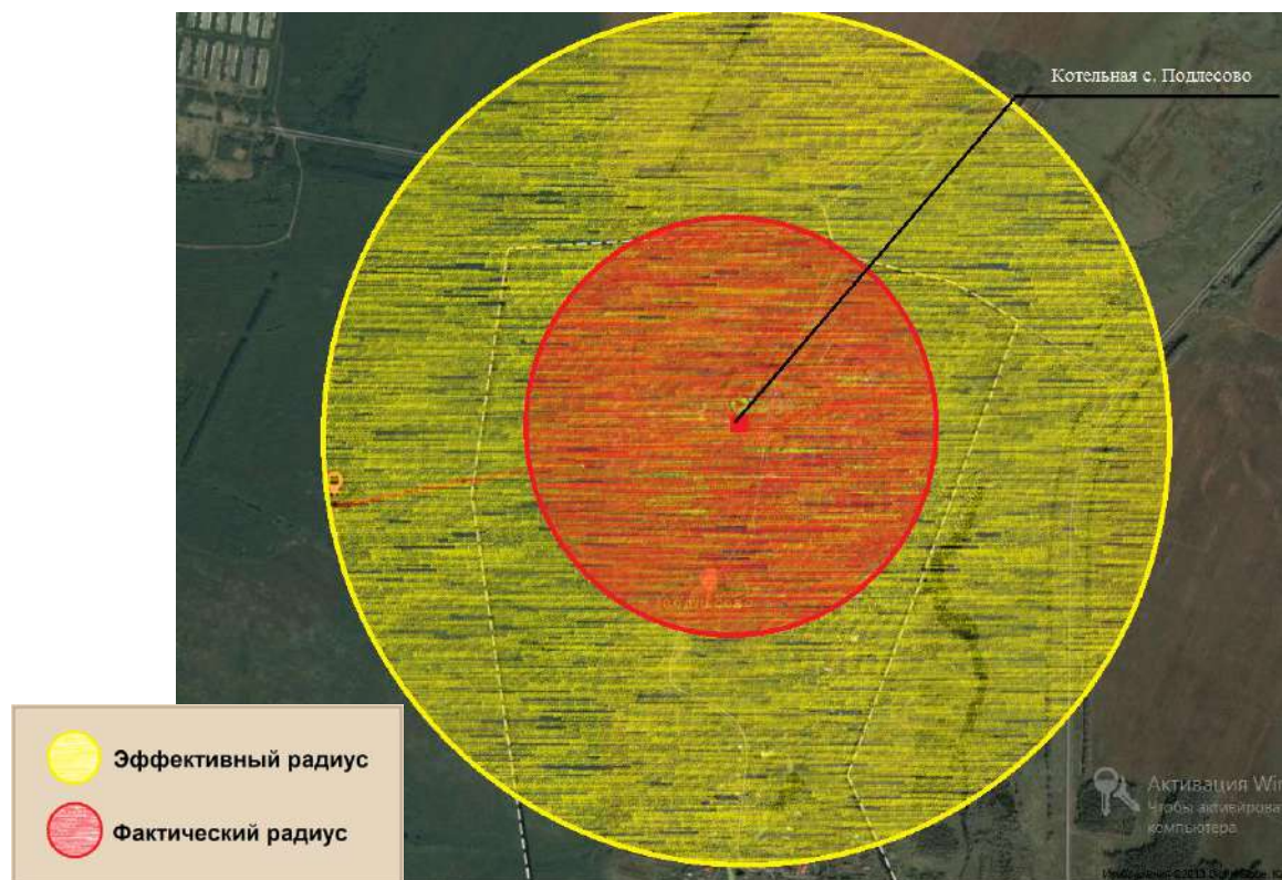
Рис. 2.1.1. Эффективный радиус теплоснабжения котельной с. Подлесово
