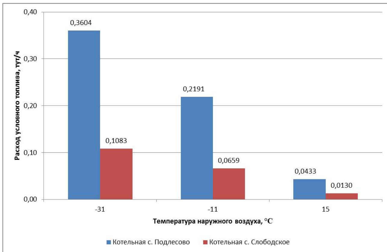
Рис. 6.2.1. Расходы основного топлива для максимального зимнего, переходного и летнего режимов работы котельных с. Подлесово и с. Слободское
