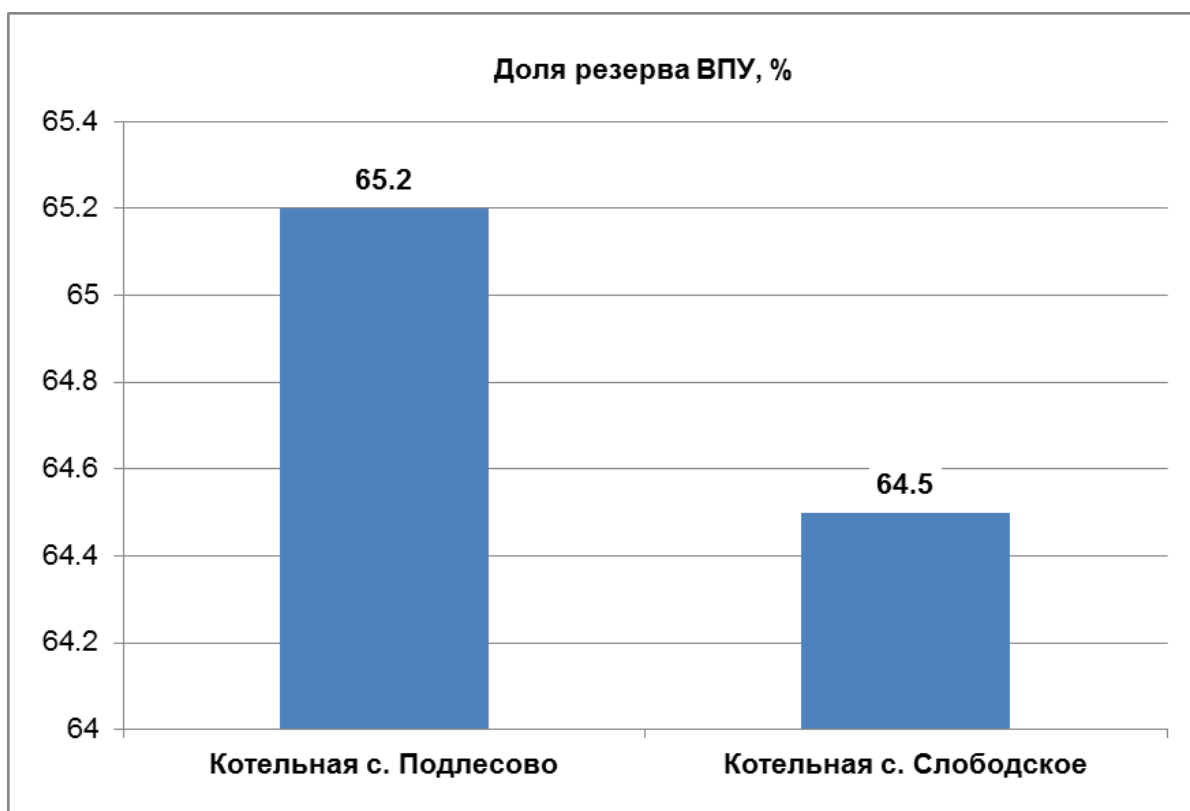
Рис. 3.1.1. Доля резерва производительности ВПУ от каждой котельной сельского поселения Слободской сельсовета
