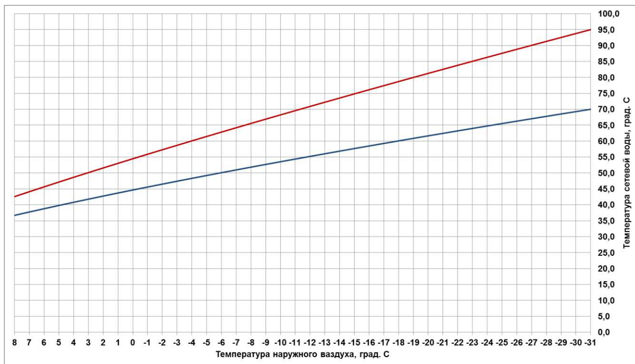
Рис. 4.2.1. Температурный график регулирования для системы теплоснабжения от котельных сельского поселения Слободской сельсовет
