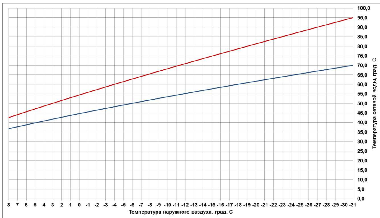
Рис. 5.8.1. Температурный график отпуска тепловой энергии от котельной МОУ СОШ с. Безводное
