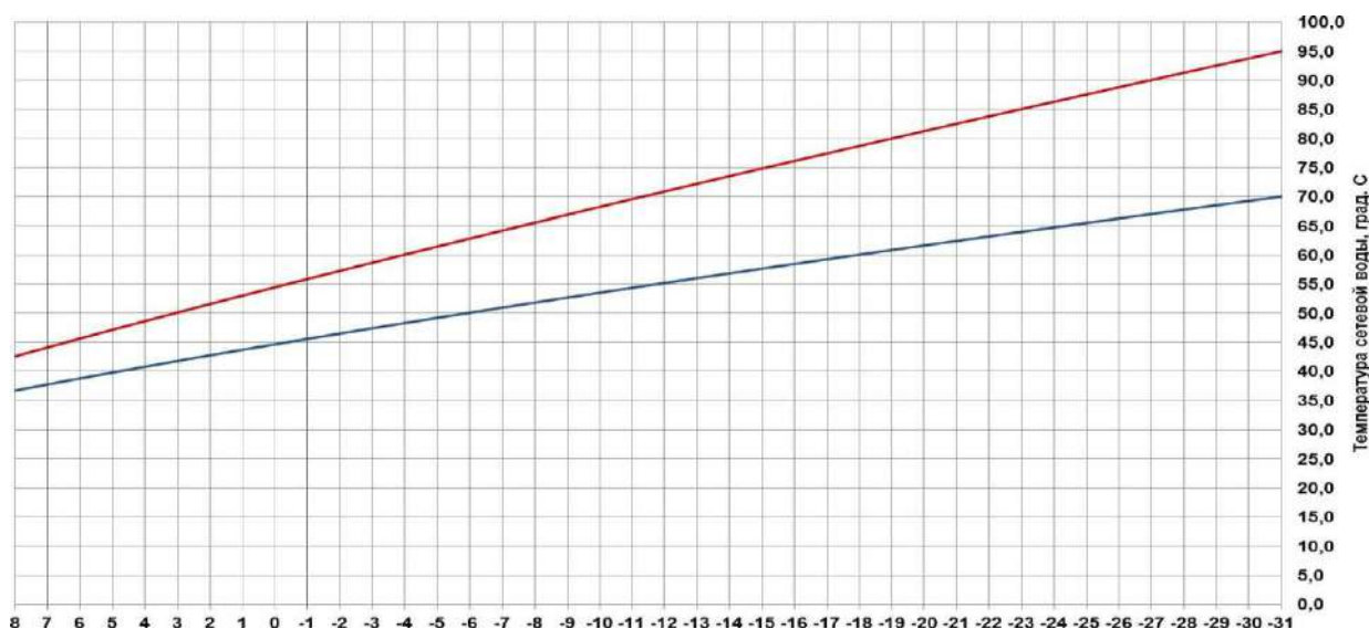
Рис. 5.8.1. Температурный график отпуска тепловой энергии от котельных д. Прокошево
