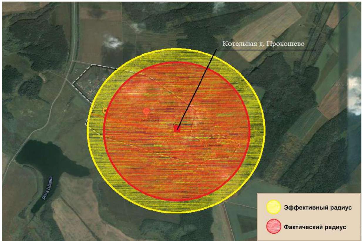
Рис. 2.5.1. Эффективный радиус теплоснабжения котельной д. Прокошево
