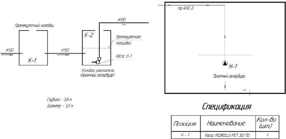
Рис. 9.1.2. Схема ФНС на ул. Котовского
