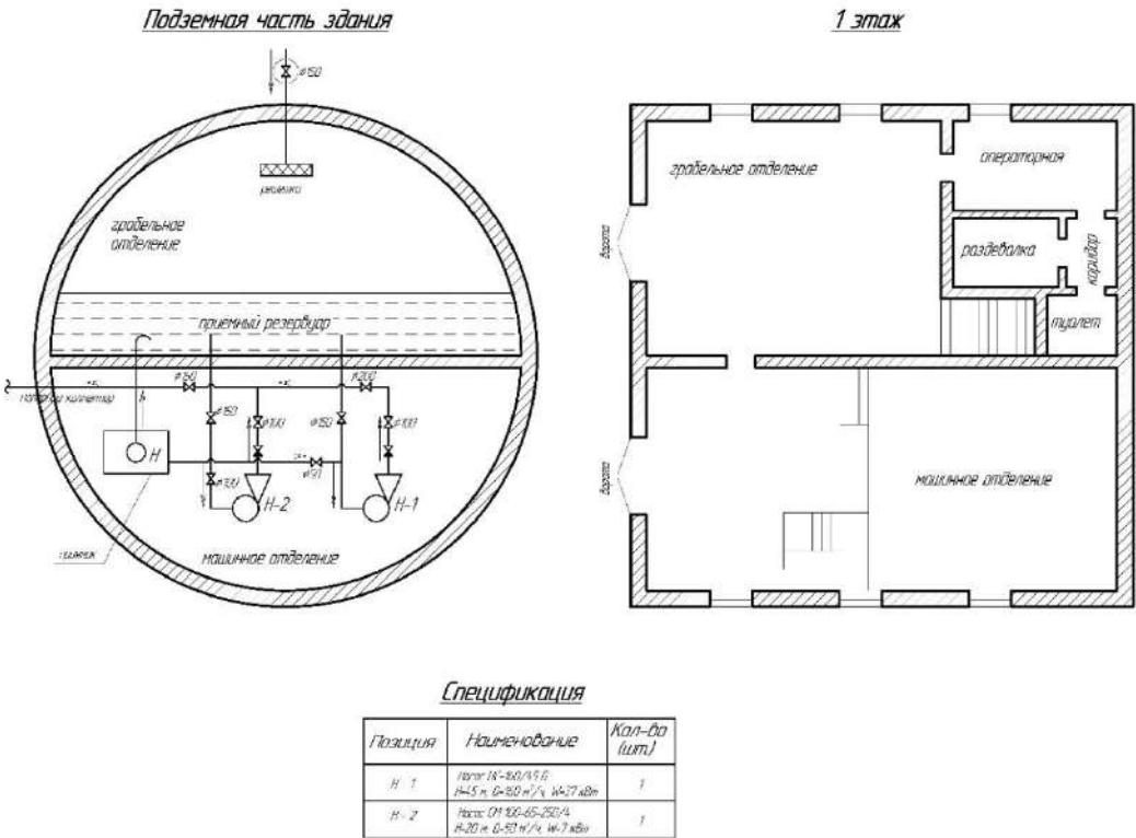
Рис. 9.1.1. Схема ФНС-5 на ул. Коминтерна
