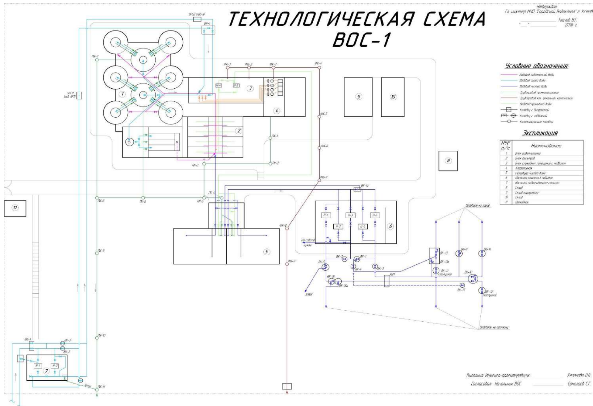
Рис. 1.3.3. Технологическая схема ВОС-1
