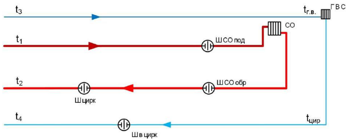
Рис. 1.5.1. Четырехтрубная схема непосредственного присоединение потребителей отопления и ГВС к тепловой сети от котельных
