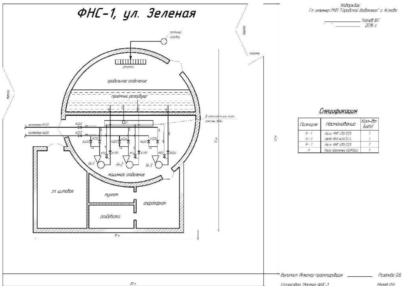
Рис. 9.1.3. Схема ФНС-1 на ул. Зеленая
